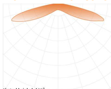
Abstrahlwinkel: 160°
