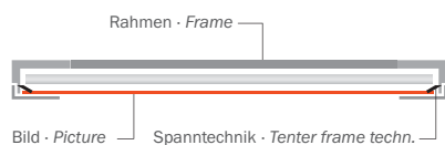
Leuchtkasten Spanntechnik mit Klapprahmen Tenter lightbox with hinged alternate frame
