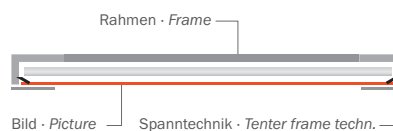
Leuchtkasten Spanntechnik mit Steckrahmen Tenter lightbox with backloading technology
